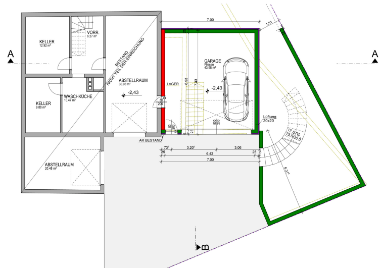
GRUNDRISS KELLERGEHÖS
