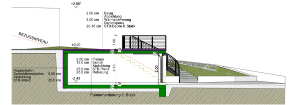
SNITT B-B
