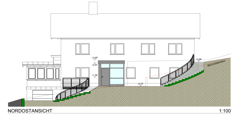
NORDOSTANSICHT
