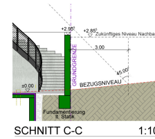
SNITT C-C
