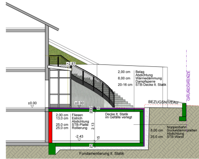
SNITT A-A
