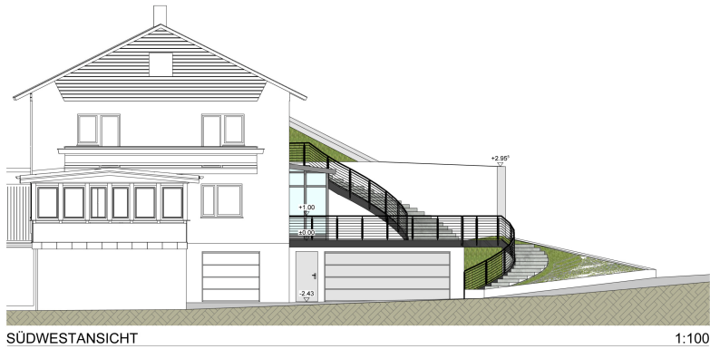
SÜDWESTANSICHT
